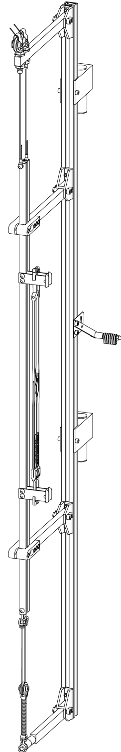
K-MAG® Dreherlitztensteuerung
