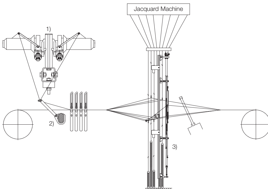
1) Klöcker Cross Leno Cone Creel 2) Klöcker Thread Reversion 3) K-MAG® Leno Heald Control
